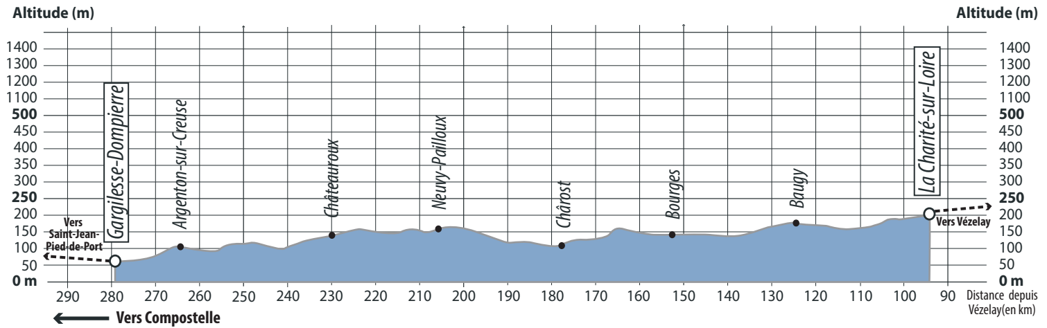
Profil topographique du chemin
