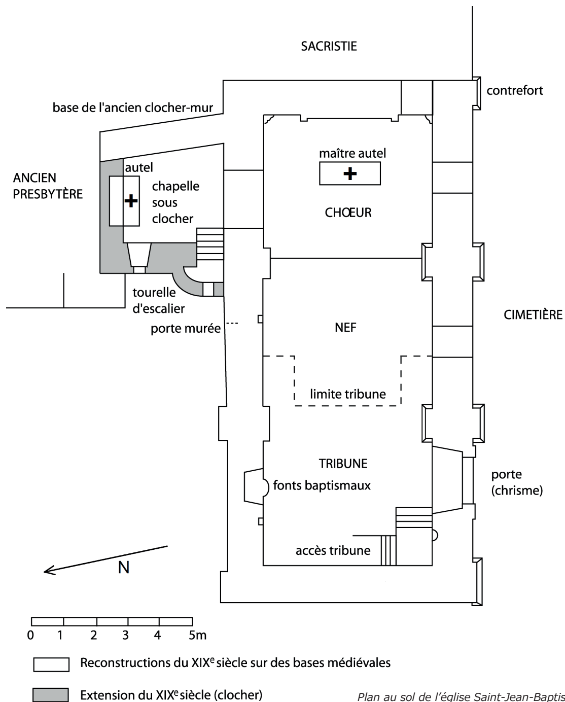
Plan au sol de l'église Saint-Jean-Baptiste de Gavarnie.
